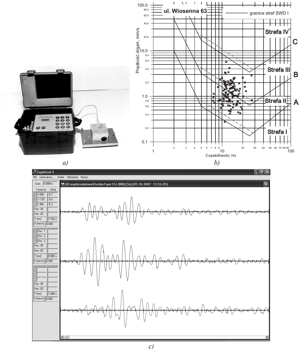
Rys. 2. Mała Stacja Monitoringu Drgań - Explo 504: a) widok ogólny; b) ocena oddziaływania z zastosowaniem skali SWD-I; c) okno dialogowe programu Explograf
